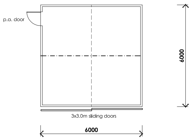
PLAN 1:100
