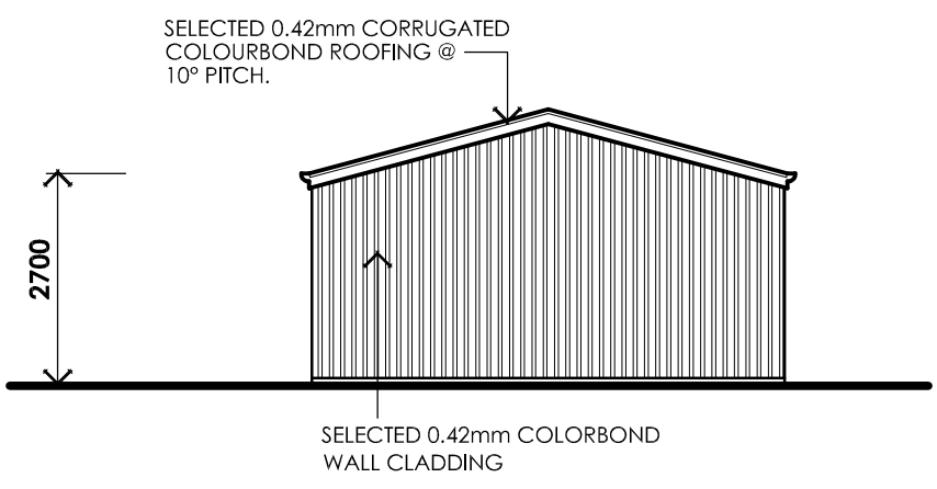
END ELEVATION 1:100
